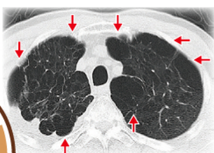
肺気腫
